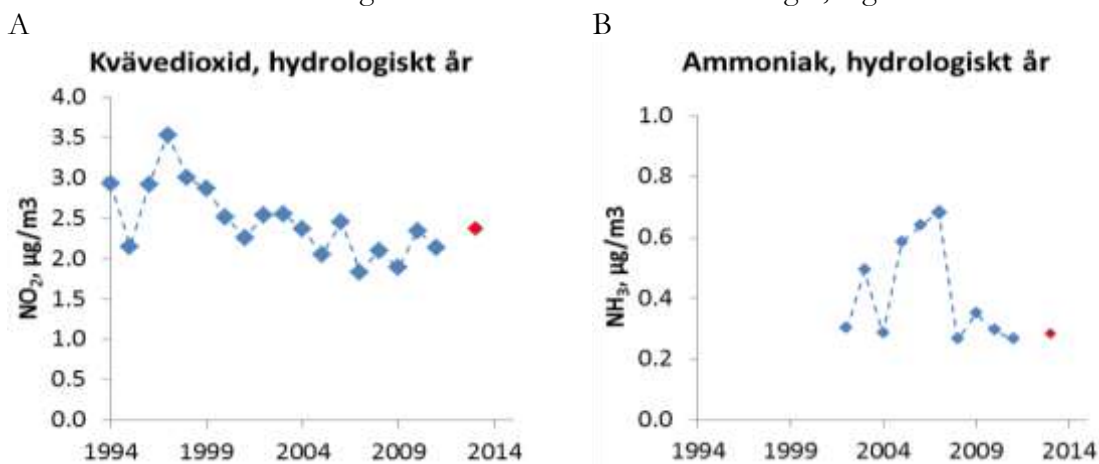
Figur 10. Lufthalter för kvävedioxid, NO 2 (A) och ammoniak, NH 3 (B) i Kvisterhult (blå markeringar) / Hjälmarsberg (röd markering).
