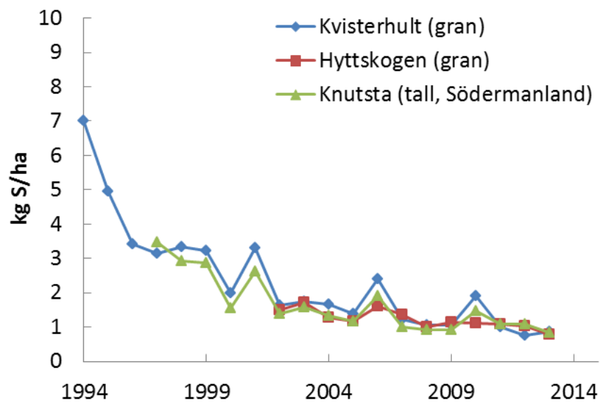
Figur 5. Svavelnedfall i granskogarna i Kvisterhult och Hyttskogen samt i tallskogen i Knutsta i Södermanlands län.
