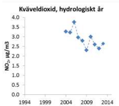
Figur B1:7. Lufthalter vid Hyttskogen (U 06) . Värden anges för kvävedioxid (NO 2 ). Vid Hyttskogen mäts även ozon som redovisas inom Ozonmättnätet i södra Sverige.
