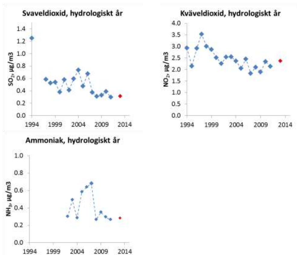
Figur B1:4. Lufthalter vid Hjälmarsberg (U 09) (röd markering) och Kvisterhult (U 04) (blå markering). Värden anges för svaveldioxid (SO 2 ), kvävedioxid (NO 2 ) och ammoniak (NH 3 ). Vid Hjälmarsberg/Kvisterhult mäts även ozon som redovisas inom Ozonmättnätet i södra Sverige.
