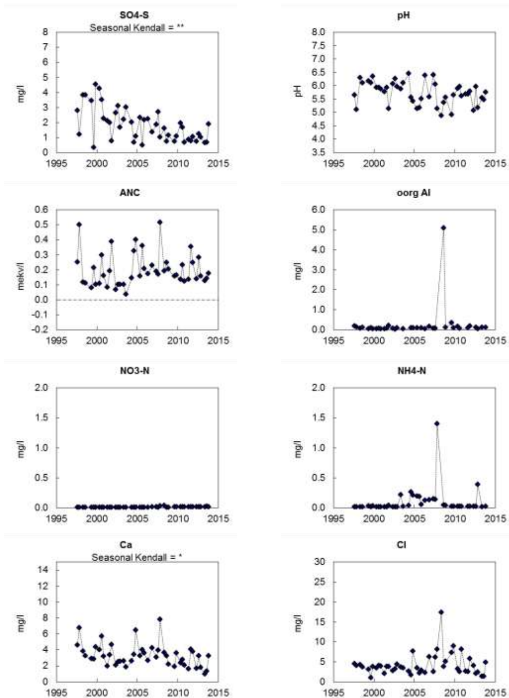
Figur B1:9. Markvattenkemi vid Knutsta, D 14 , i Södermanlands län. Sulfatsvavel (SO 4 -S); pH; markvattnets syraneutraliserande förmåga (ANC); oorganiskt aluminium (oorg Al); nitratkväve (NO 3 -N); ammoniumkväve (NH 4 -N); kalciumhalt (Ca 2+ ) och klorid (Cl). Saknade värden innebär oftast att marken varit för torr. Trendanalys har genomförts med hjälp av Seasonal-Kendall metodik och signifikansnivåer anges, ovanför respektive diagram, i de fall där signifikanta trender påvisats. Observera att olika skalor mot lokalerna i Västmanlands län kan förekomma.
