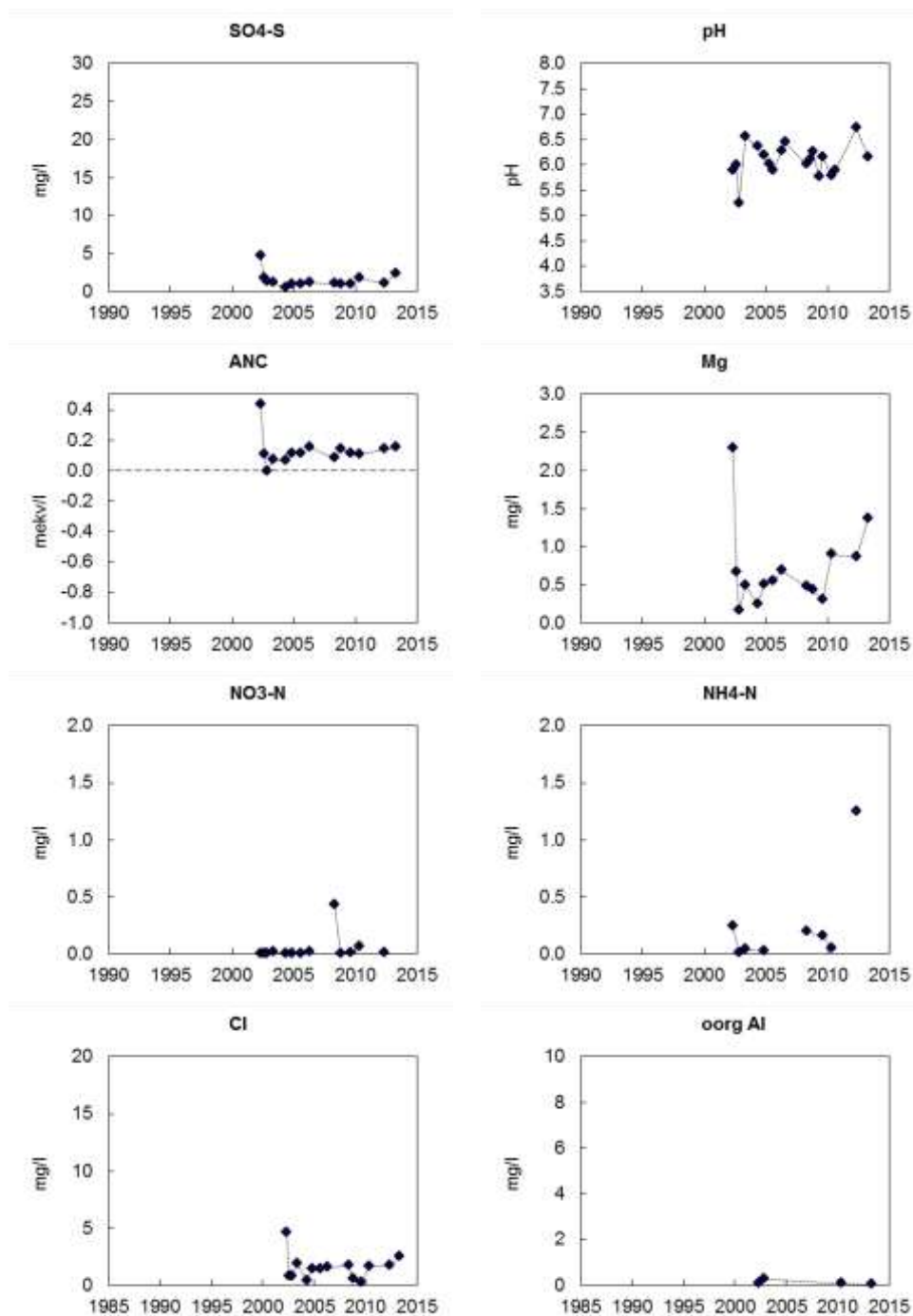
Figur B1:6. Markvattenkemi vid Hyttskogen, U 06: sulfatsvavel ( \text{SO}_4\text{-S} ); pH; markvattnets syra-neutraliserande förmåga (ANC); magnesiumhalt ( \text{Mg}^{2+} ); nitratkväve ( \text{NO}_3\text{-N} ); ammoniumkväve ( \text{NH}_4\text{-N} ); klorid (Cl) och oorganiskt aluminium (oorg Al). Saknade värden innebär oftast att marken varit för torr. Trendanalys har genomförts med hjälp av Seasonal-Kendall och signifikansnivåer anges, ovanför respektive diagram, i de fall där signifikanta trender påvisats.
