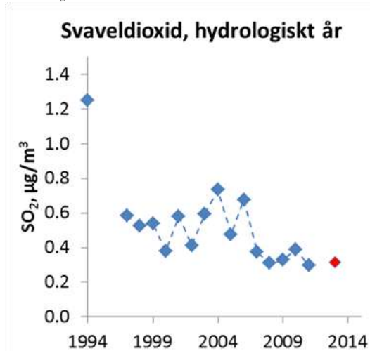
Figur 4. Svaveldioxidhalter i luften i Kvisterhult (blå symbol) / Hjälmarsberg (röd symbol) i södra delen av Västmanlands län.
