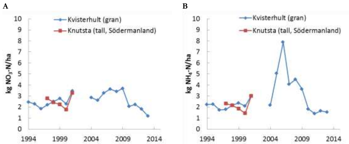
Figur 11. Årliga värden för nedfall av nitratkväve (A) och ammoniumkväve (B) med nederbörden till öppet fält till Kvisterhult i Västmanlands län samt Knutsta i Södermanlands län. Nedfallet är summerat som hydrologiskt år (okt-sept).
