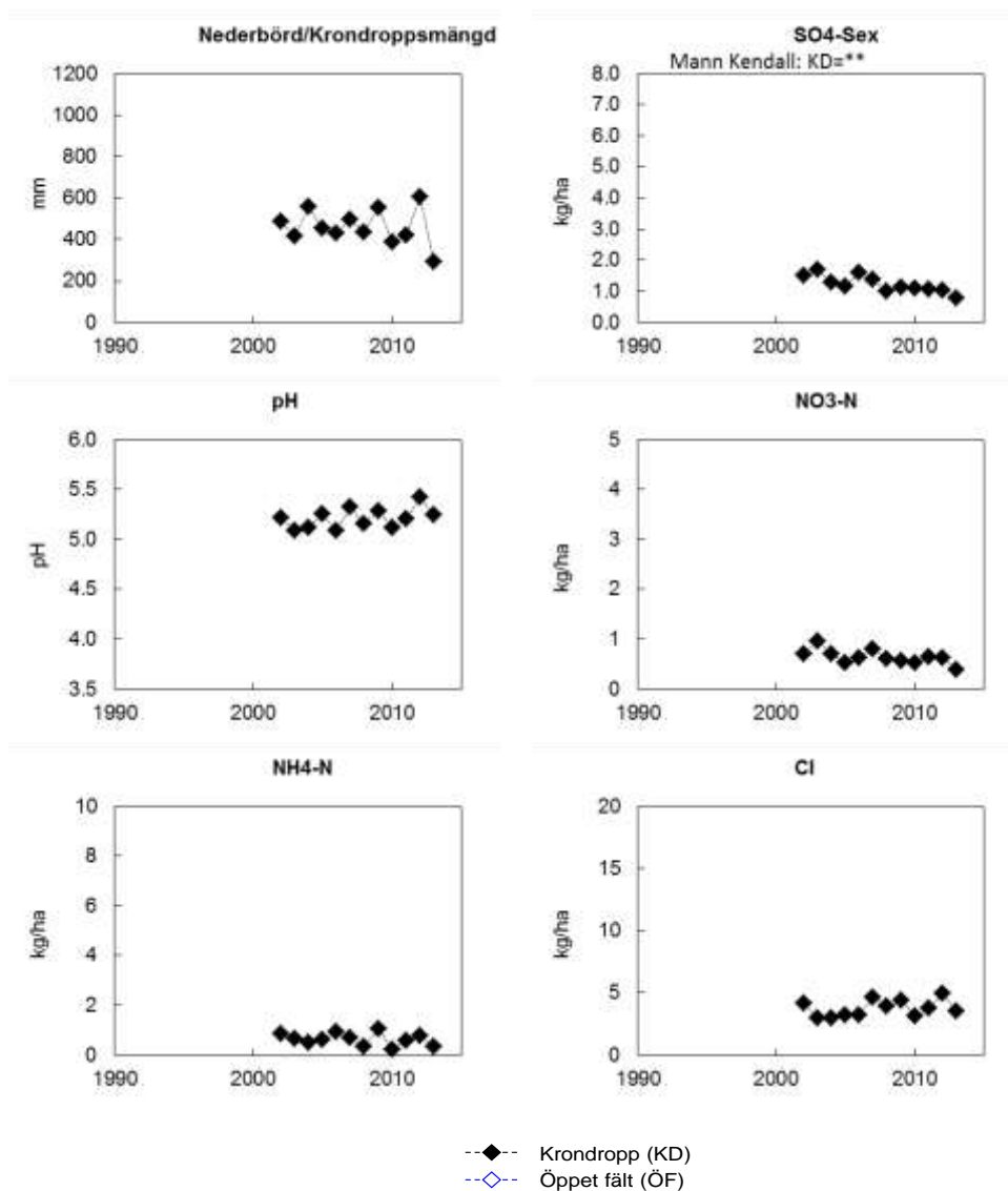
Figur B1:5. Årliga värden (hydrologiskt år) för depositionen i krondropp och över öppet fält vid Hyttskogen, U 06. I figuren visas uppmätt nederbörd över öppet fält samt krondroppsmängder, uttryckt som mm. Deposition redovisas sedan mätningarna påbörjades för ett urval av ämnen: sulfatsvavel utan havssaltsbidrag (SO 4 -S ex); pH; nitratkväve (NO 3 -N); ammoniumkväve (NH 4 -N) och kloridjoner (Cl). ÖF, öppet fält; KD, krondropp. Trendanalys har genomförts med hjälp av Mann-Kendall analys och signifikansnivåer anges, ovanför respektive diagram, i de fall där signifikanta trender påvisats.
