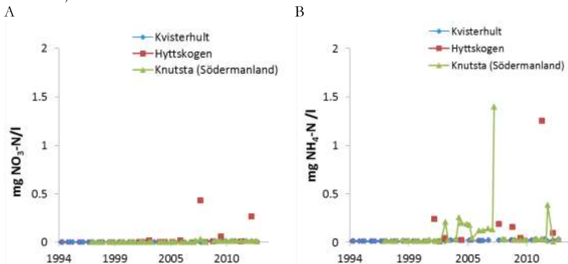
Figur 13. Halterna i markvattnet på 50 cm djup vid olika platser i Västmanlands län samt Södermanlands län av nitratkväve (NO 3 -N) (A) samt halterna av ammoniumkväve (NH 4 -N) (B). Inga förändringar är statistiskt säkerställda.
