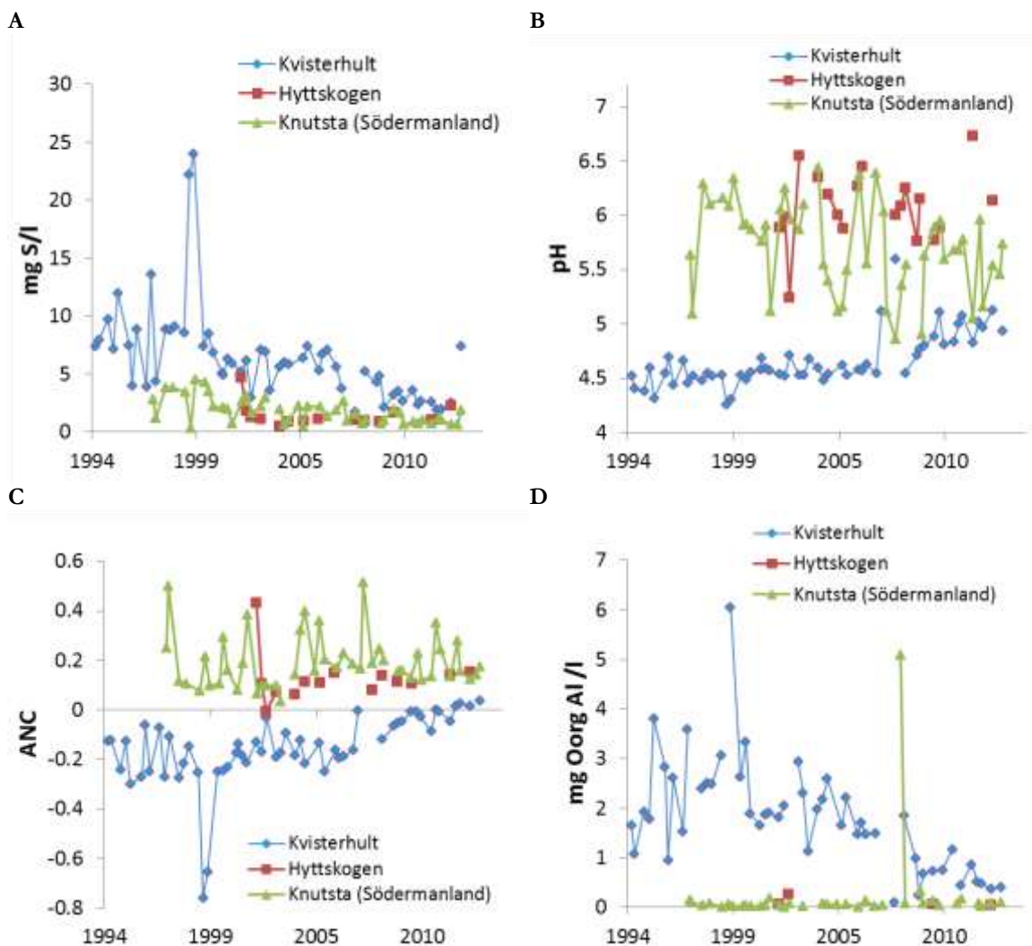
Figur 7. Halterna av sulfatsvavel (A, \text{SO}_4\text{-S} ), pH (B), syraneutraliserande förmåga (C, ANC) och halten oorganiskt aluminium (D, oorg-Al) i markvattnet på 50 cm djup vid olika platser i Västmanlands samt Södermanlands län, uppmätt inom Krondropps nätet. Följande förändringar är statistiskt säkerställda: \text{SO}_4\text{-S} har minskat signifikant vid Kvisterhult och Knutsta (Södermanland); pH och ANC har ökat signifikant vid Kvisterhult och oorg-Al har minskat signifikant vid Kvisterhult.
