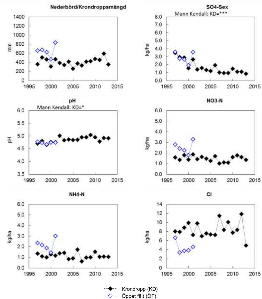
Figur B1:8. Årliga värden (hydrologiskt år) för depositionen via krondropp och över öppet fält vid Knutsta, D 14 , i Södermanlands län. I figuren visas uppmätt nederbörd över öppet fält samt krondroppsmängder, uttryckt som mm. Deposition redovisas sedan mätningarna påbörjades för ett urval av ämnen: sulfatsvavel utan havssaltsbidrag (SO 4 -S ex); pH; nitratkväve (NO 3 -N); ammoniumkväve (NH 4 -N) och kloridjoner (Cl). ÖF, öppet fält; KD, krondropp. Trendanalys har genomförts med hjälp av Mann-Kendall metodik och signifikansnivåer anges, ovanför respektive diagram, i de fall där signifikanta trender påvisats. Observera att olika skalor mot lokalerna i Västmanlands län kan förekomma.
