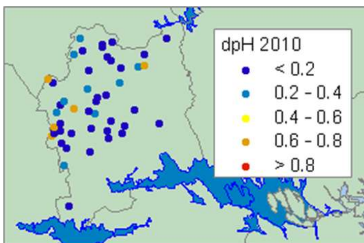
Figur 9. pH-förändring sedan förindustriell tid (dpH) i sjöar 2010, baserat på MAGIC-biblioteket. En sjö räknas som antropogent försurad om pH som årsmedian har sjunkit med minst 0,4 enheter sedan förindustriell tid (dpH > 0,4), vilket markeras med gula, orange och röda symbolerna på kartan. Analysen inkluderar kalkade försurade sjöar, där vattenkemin i frånvaro av kalkning beräknats. Källa: Fölster & Valinia, (2012).
