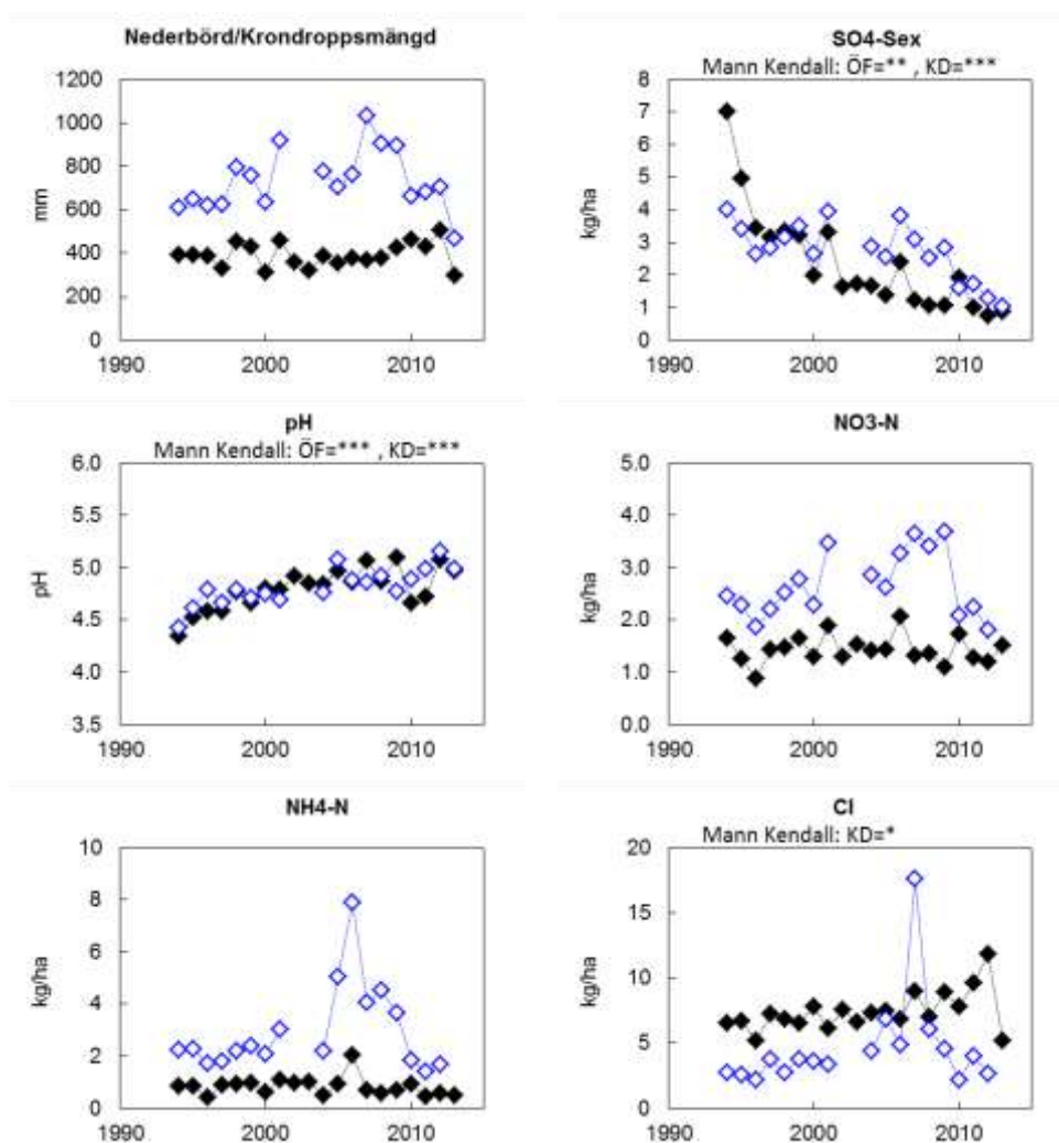
Figur B1:2. Årliga värden (hydrologiskt år) för depositionen i krondropp och över öppet fält vid Kvisterhult, U 04 . I figuren visas uppmätt nederbörd över öppet fält samt krondroppsmängder, uttryckt som mm. Deposition sedan mätningarna påbörjades redovisas för ett urval av ämnen: sulfatsvavel utan havssaltsbidrag (SO 4 -S ex); pH; nitratkväve (NO 3 -N); ammoniumkväve (NH 4 -N) och kloridjoner (Cl - ). ÖF, öppet fält; KD, krondropp. Trendanalys har genomförts med hjälp av Mann-Kendall analys och signifikansnivåer anges, ovanför respektive diagram, i de fall där signifikanta trender påvisats.
