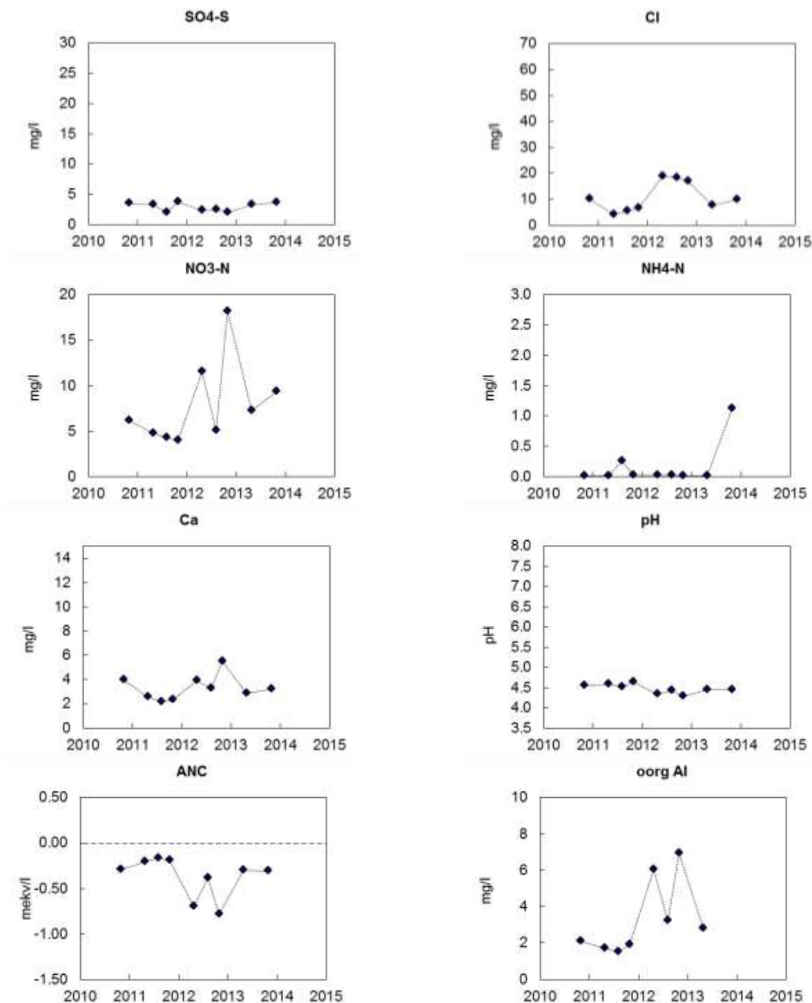
Figur B1:17. Markvattenkemi vid Stenshult, M 16: sulfatsvavel (SO 4 -S), kloridhalt (Cl), nitratkväve (NO 3 -N), ammoniumkväve (NH 4 -N), kalciumhalt (Ca 2+ ), pH, markvattnets syraneutraliserande förmåga (ANC) och oorganiskt aluminium (oorg Al). Saknade värden innebär oftast att marken varit för torr. Trendanalys har genomförts med hjälp av Seasonal-Kendall och signifikansnivåer anges ovanför respektive diagram, i de fall där signifikanta trender påvisats.
