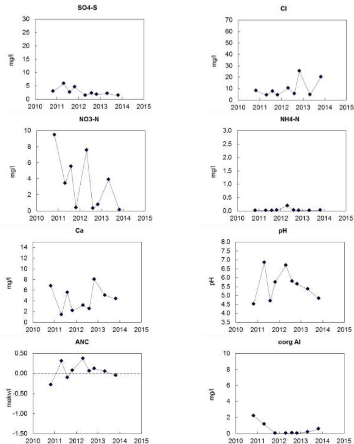
Figur B1:20. Markvattenkemi vid Baldringe, M 17 : sulfatsvavel (SO 4 -S), kloridhalt (Cl), nitratkväve (NO 3 -N), ammoniumkväve (NH 4 -N), kalciumhalt (Ca 2+ ), pH, markvattnets syraneutraliserande förmåga (ANC) och oorganiskt aluminium (oorg Al). Sknade värden innebär oftast att marken varit för torr. Trendanalys har genomförts med hjälp av Seasonal-Kendall och signifikansnivåer anges ovanför respektive diagram, i de fall där signifikanta trender påvisats.
