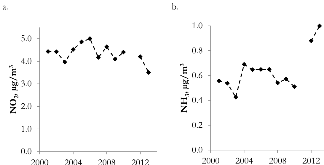
Figur 4. Lufthalter för kvävedioxid, NO 2 (a) och ammoniak, NH 3 (b) i Västra Torup/Hissmossa. Halterna från 2001 till 2010 är från Västra Torup, medan de två senaste årens mätningar är från Hissmossa.
