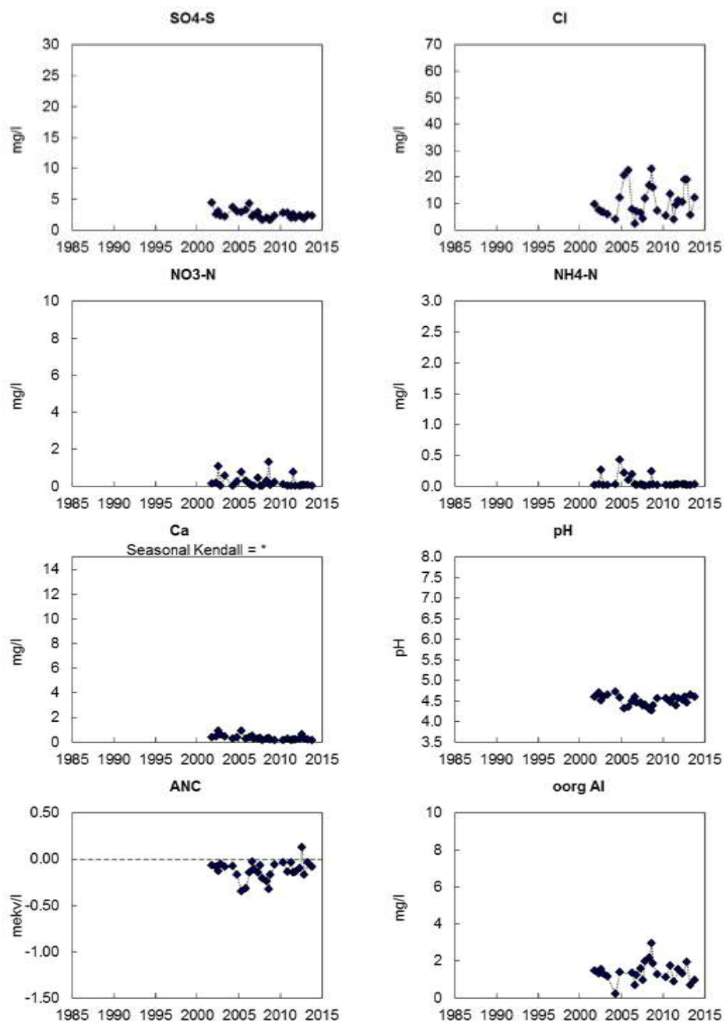
Figur B1:9. Markvattenkemi vid Maryd, L 15 : sulfatsvavel (SO 4 -S), kloridhalt (Cl), nitratkväve (NO 3 -N), ammoniumkväve (NH 4 -N), kalciumhalt (Ca 2+ ), pH, markvattnets syranneutraliserande förmåga (ANC) och oorganiskt aluminium (oorg Al). Sknade värden innebär oftast att marken varit för torr. Trendanalys har genomförts med hjälp av Seasonal-Kendall och signifikansnivåer anges ovanför respektive diagram, i de fall där signifikanta trender påvisats.
